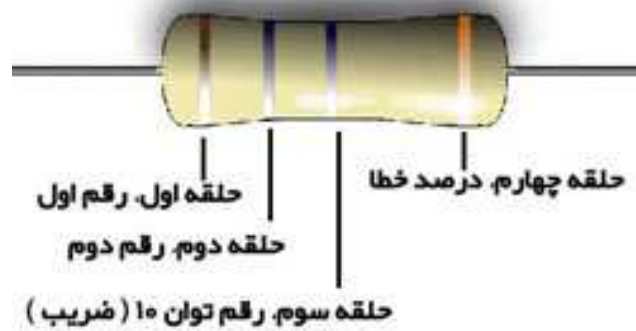
نمایش مقاومت بر روی برد چاپی
